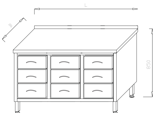
Stół z 9 szufladami ML 01.15
