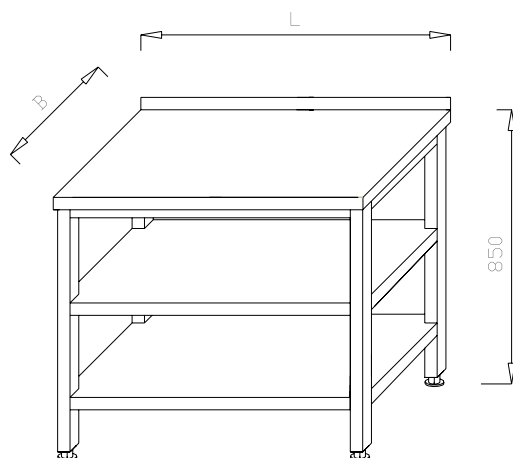
Stół z szafką ML 01.05
