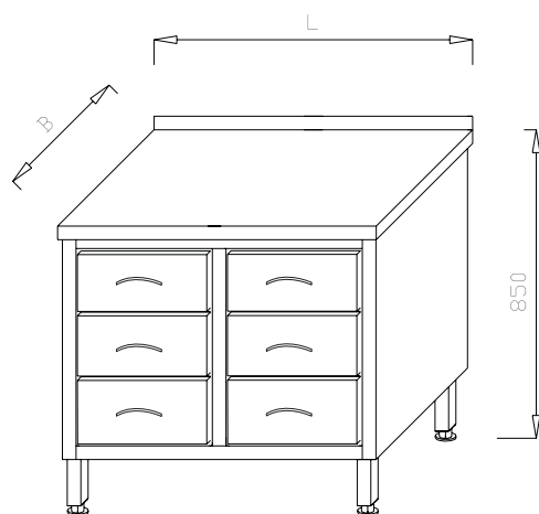
Stół z 6 szufladami ML 01.14
