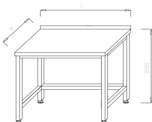
Stół przyścienny ML 01.02
