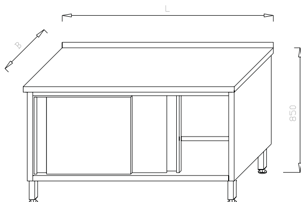
Stół z blokiem 3 szuflad ML 01.06
