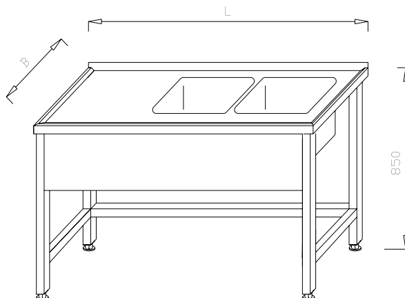
Stół ze zlewem 2-komorowym ML 02.05
