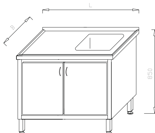
Stół ze zlewem 1-komorowym i szafką ML 02.03
