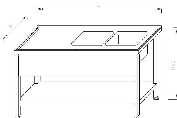
Stół ze zlewem 2-komorowym i półką ML 02.06
