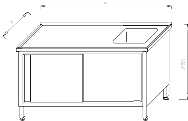
Stół ze zlewem 1-komorowym i szafką ML 02.04
