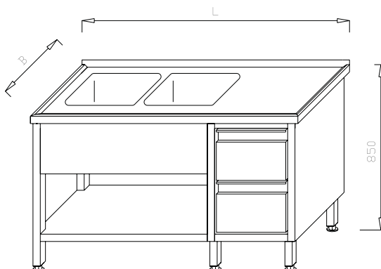
Stół ze zlewem 2-komorowym, szufladami i półką KL 02.13
