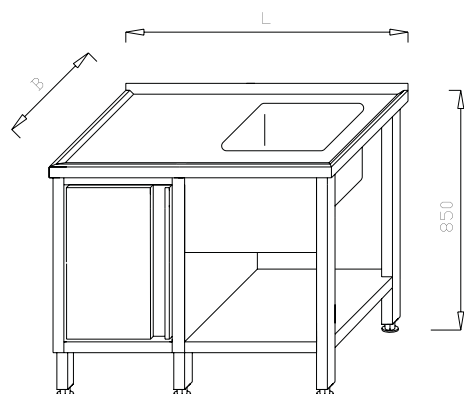
Stół ze zlewem 1-komorowym, szafką i półką KL 02.12
