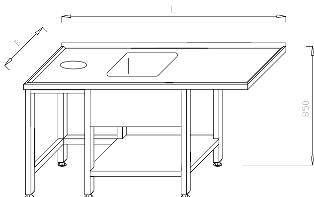
Stół ze zlewem 1-komorowym, otworem i półką KL 02.08
