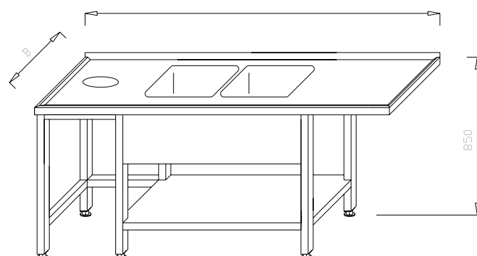
Stół ze zlewem 2-komorowym, otworem i półką KL 02.09
