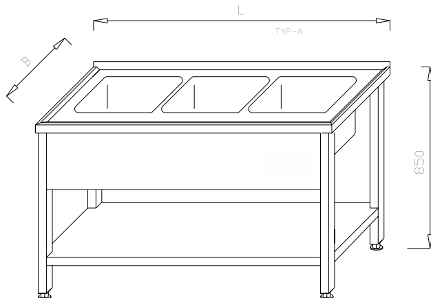
Stół ze zlewem 3-komorowym i półką KL 02.16
