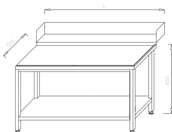
Stół wyładowniczy do zmywarek KL 02.21
