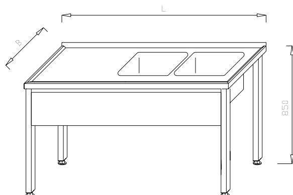
Stół ze zlewem 2-komorowym KL 02.05
