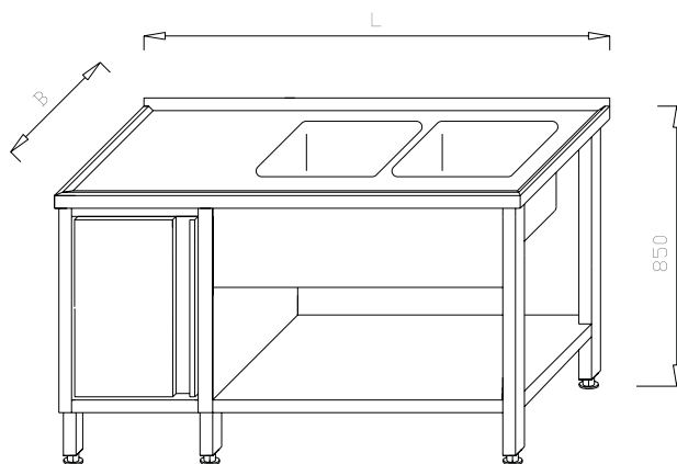
Stół ze zlewem 2-komorowym, szafką i półką KL 02.10
