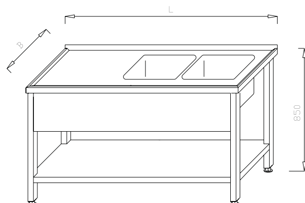
Stół ze zlewem 2-komorowym i półką KL 02.06
