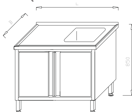
Stół ze zlewem 1-komorowym i szafką KL 02.03
