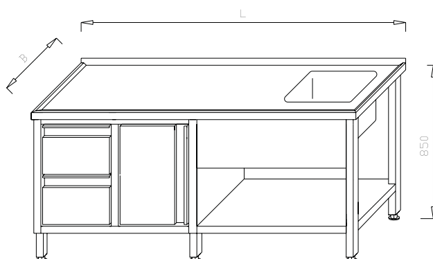
Stół ze zlewem 1-komorowym, szafką, szufladami i półką KL 02.11
