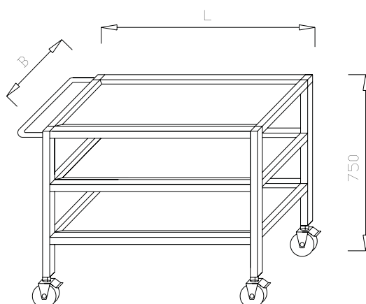
Wózek transportowy KL 04.03
