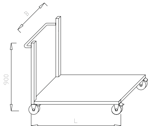
Wózek transportowy KL 04.01
