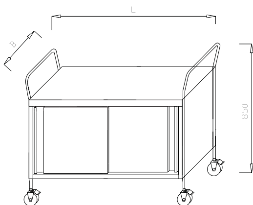
Wózek z szafką KL 04.05
