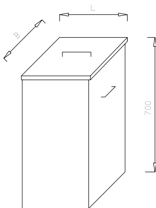
Pojemnik na odpadki KL 04.08
