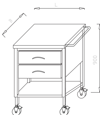
Asystor z 2 szufladami i półką ML 04.07
