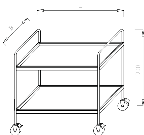
Stolik jezdny z półką ML 04.01
