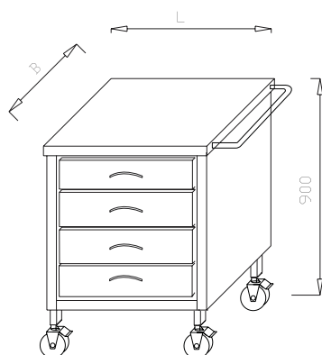
Asystor z 4 szufladami ML 04.05
