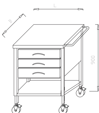
Asystor z 3 szufladami i półką ML 04.08
