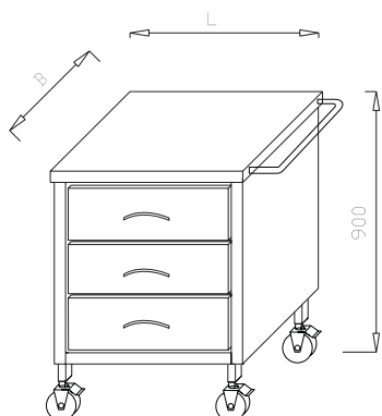
Asystor z 3 szufladami ML 04.04
