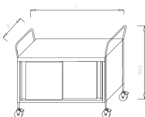
Stolik jezdny z szafką ML 04.03
