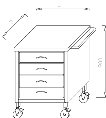
Asystor z 4 szufladami SL 01.24
