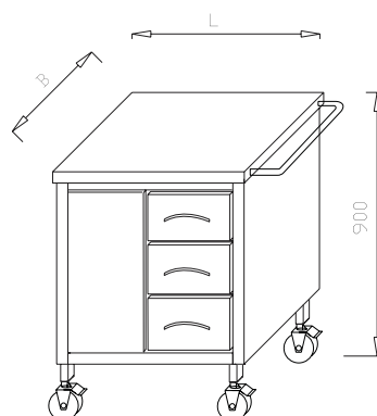
Asystor z 3 szufladami i szafką SL 01.26
