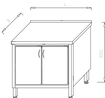
Stół z szafką, drzwi na zawiasie SL 01.06
