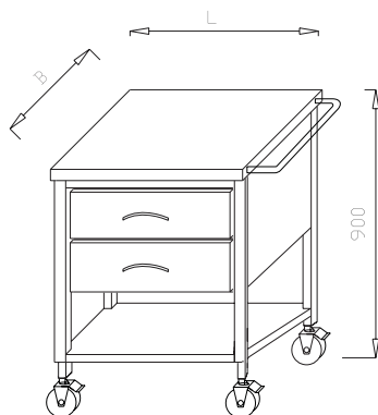
Asystor z 2 szufladami i półką SL 01.21
