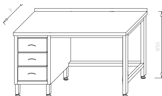
Biurko - stół z blokiem 3 szuflad SL 01.13
