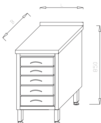
Stół - blok 5 szuflad SL 01.05
