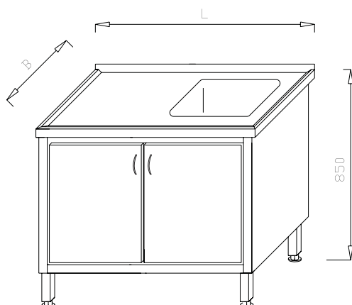
Stół ze zlewem 1-komorowym i szafką SL 01.15
