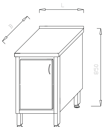
Stół - szafka, drzwi na zawiasie SL 01.01
