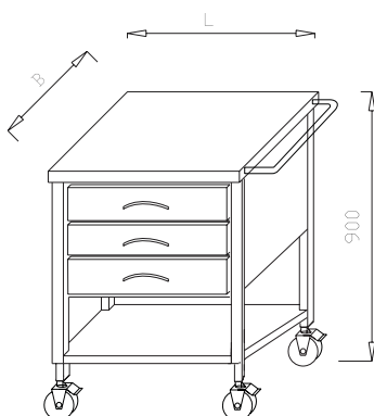
Asystor z 3 szufladami i półką SL 01.22
