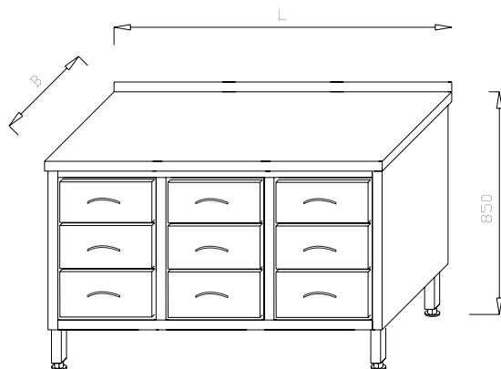
Stół - blok 9 szuflad SL 01.10
