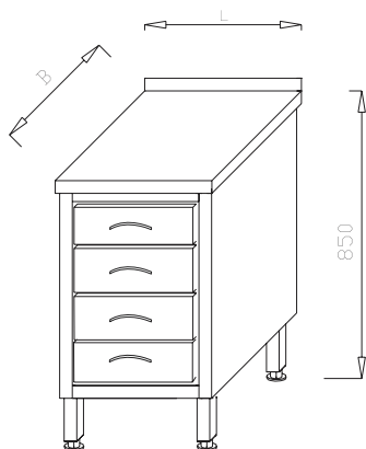
Stół - blok 4 szuflad SL 01.04
