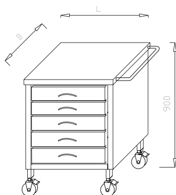
Asystor z 5 szufladami SL 01.25
