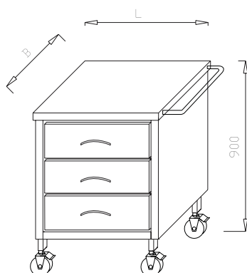
Asystor z 3 szufladami SL 01.23
