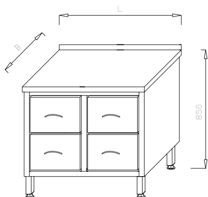
Stół - blok 4 szuflad SL 01.07
