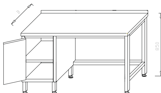
Biurko - stół z szafką SL 01.14
