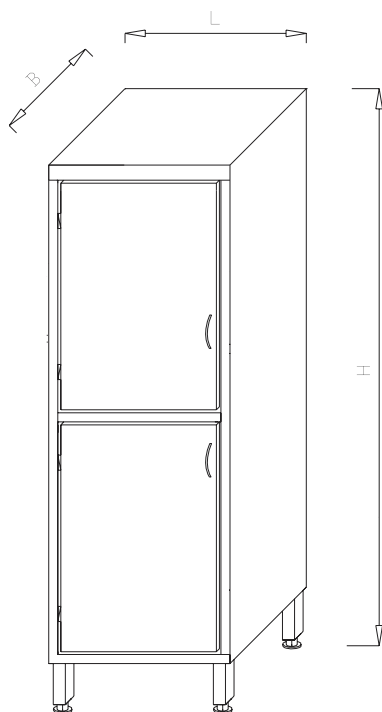
Szafa pojedyncza, drzwi na zawiasie dzielone SL 01.19
